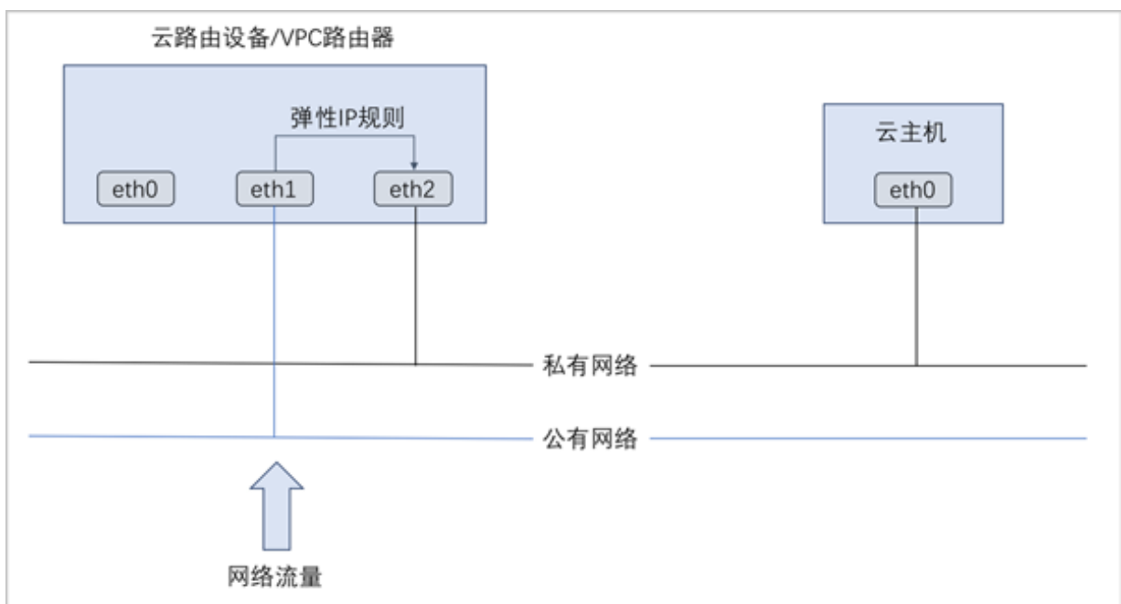
图 329: 云路由网络/VPC下弹性IP的应用场景
