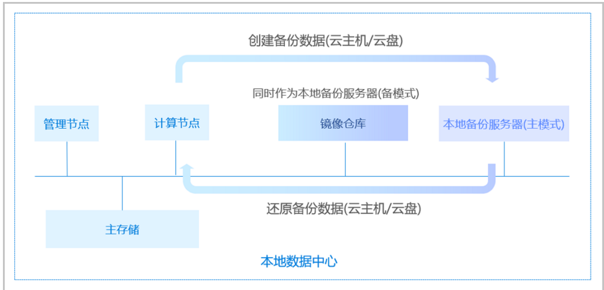
图 969: 本地灾备场景2
