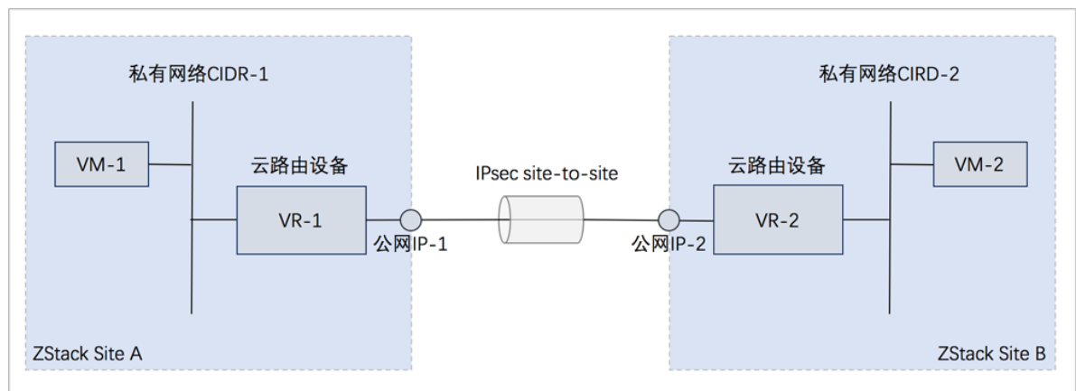
图 351: 云路由网络下IPsec隧道应用场景
