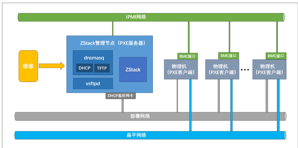
图 888: 裸金属管理原理图
